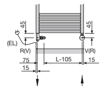
монтаж для работы в смешанном режиме
