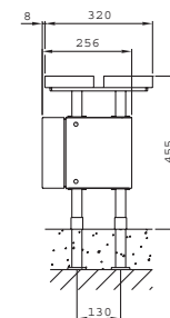
4-трубная модель
